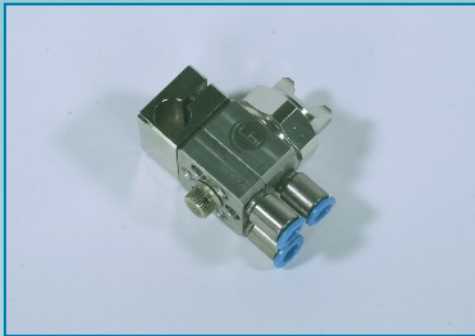
LB-002 mit Flachstrahldüse und Anzeigeschraube mit Knopf
