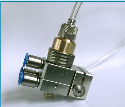
LB-002 mit Koaxial Adapter und Mini-Sprühdüse
